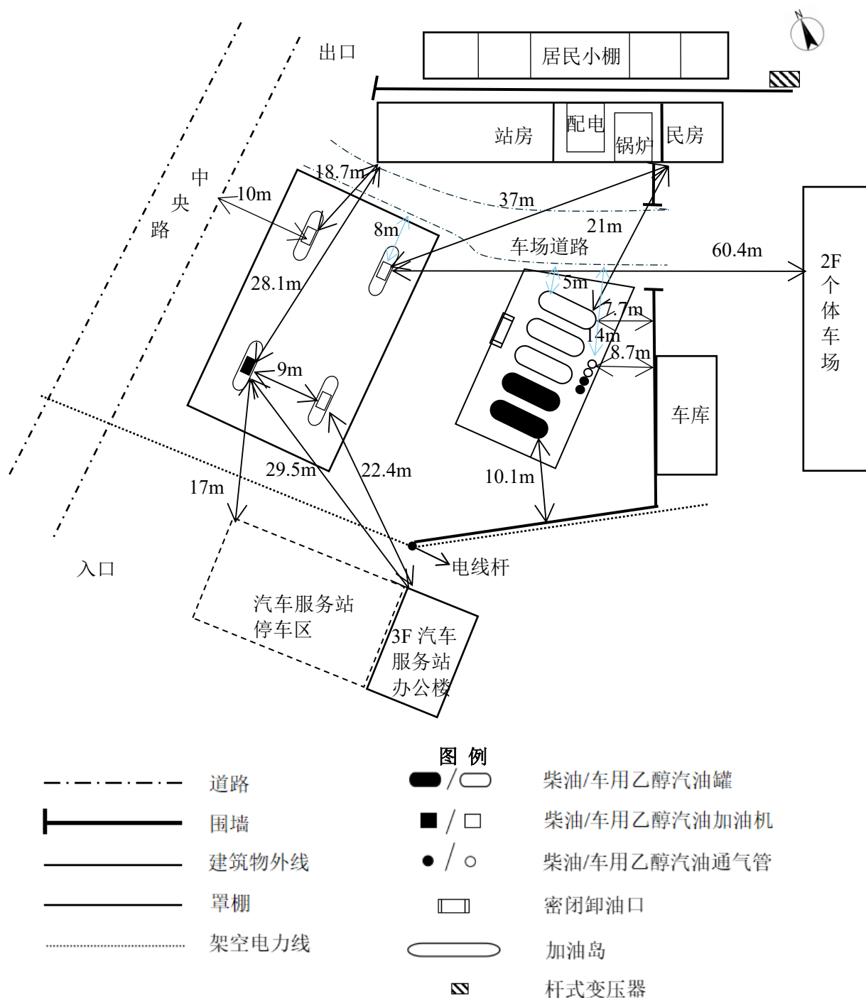
图 2.7.2-1 平面布置图
