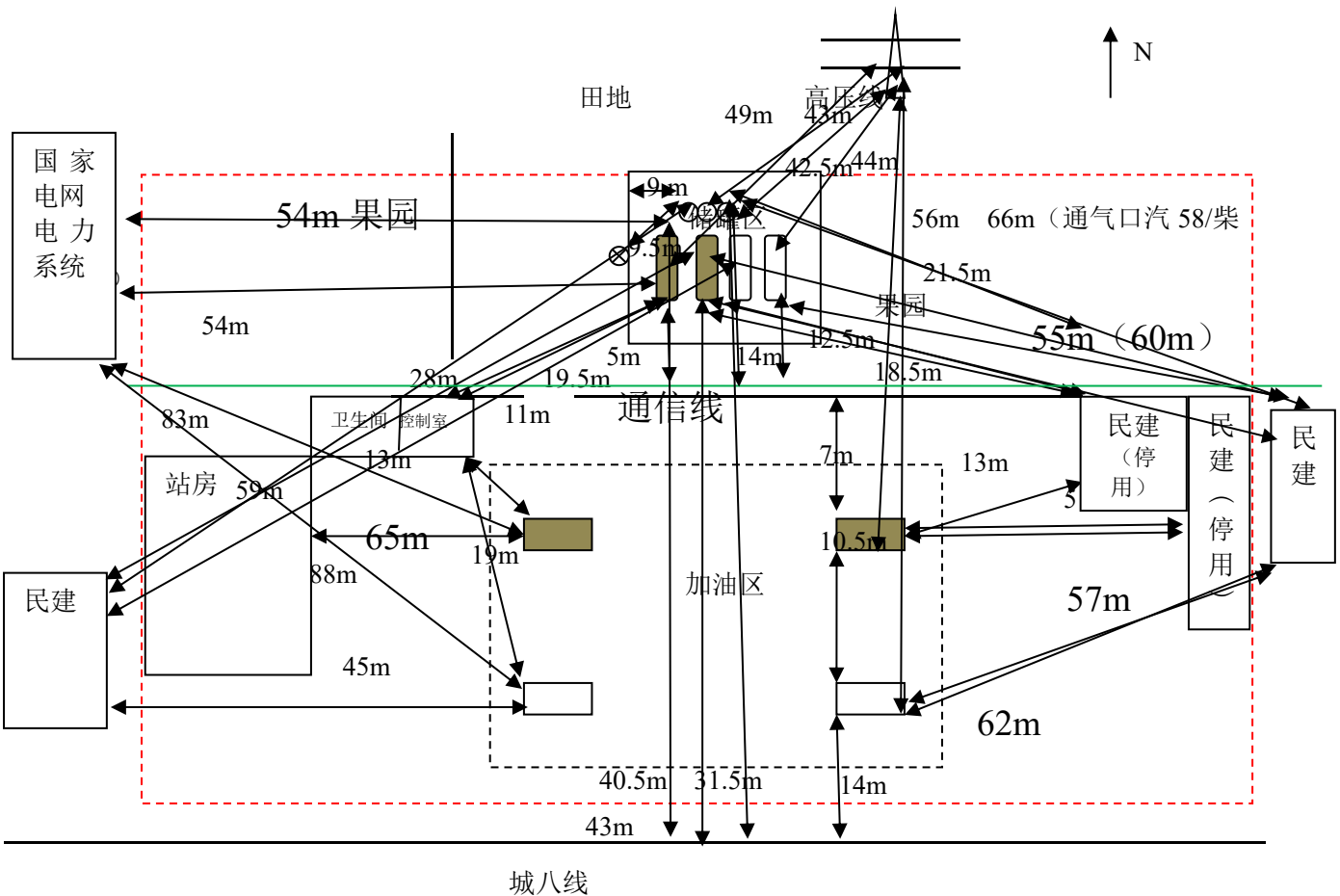
图 2.7.2-1 平面布置图
