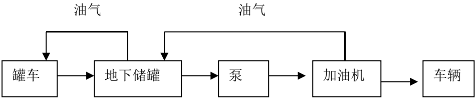
图 2.4.1 卸油、加油工艺流程图
