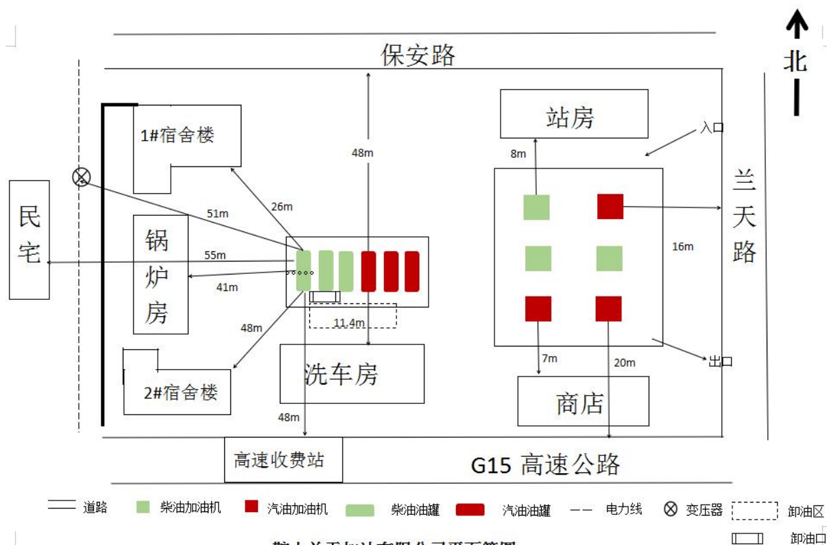
鞍山蓝天加油有限公司平面简图
