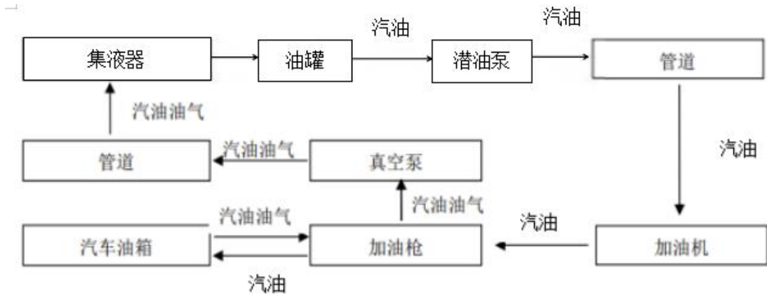
图 2.4.1-3 乙醇汽油加油及油气回收工艺流程图
