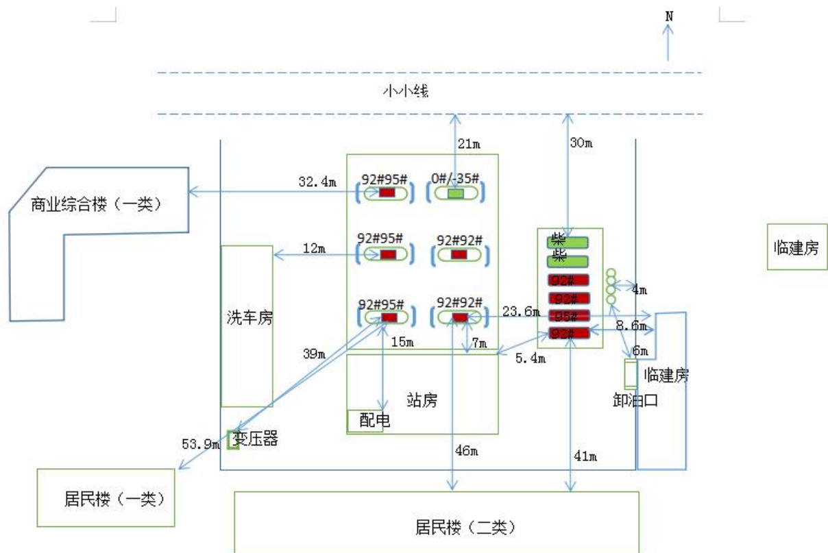
灯塔市运输公司加油站平面示意图
