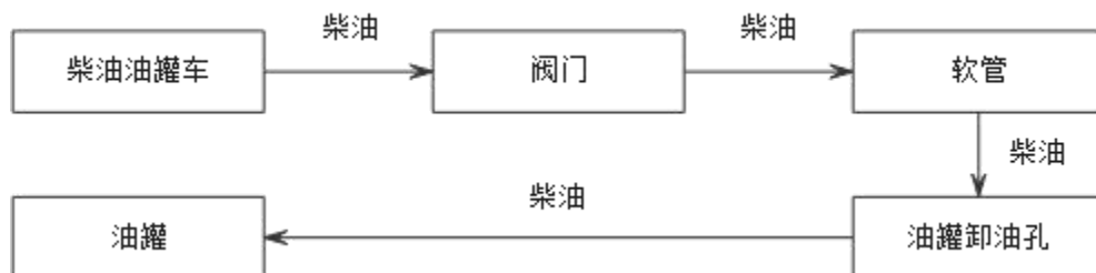
图 2.4.1-2 柴油罐车密闭卸油工艺流程图
