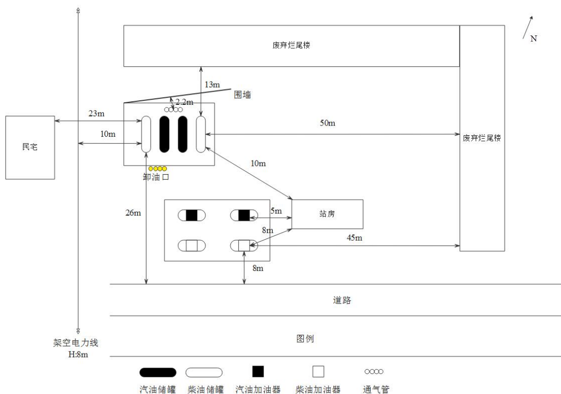
图 2.7.2-1 平面布置图
