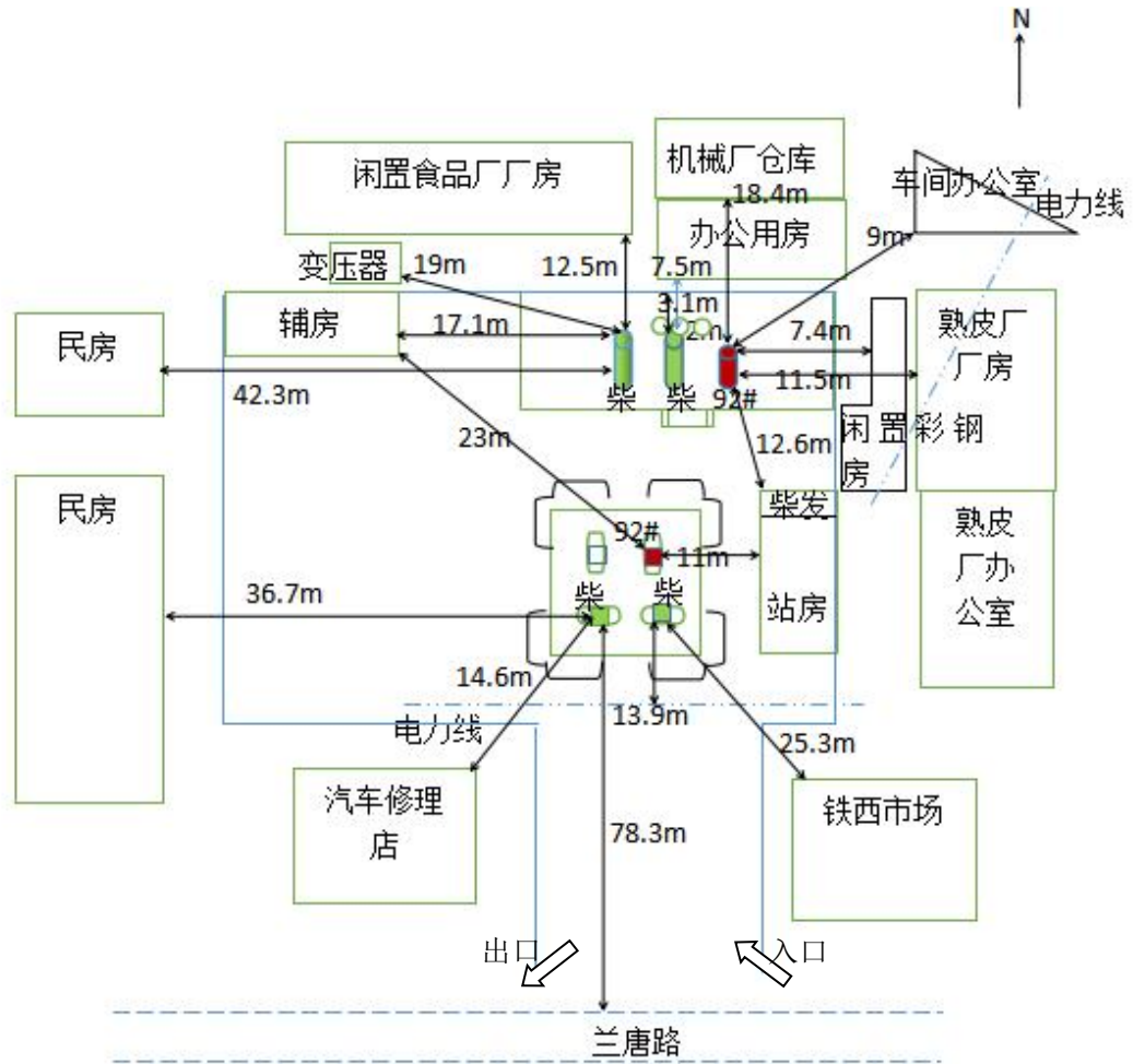
辽阳县首山供销合作社农机油供应站平面示意简图
